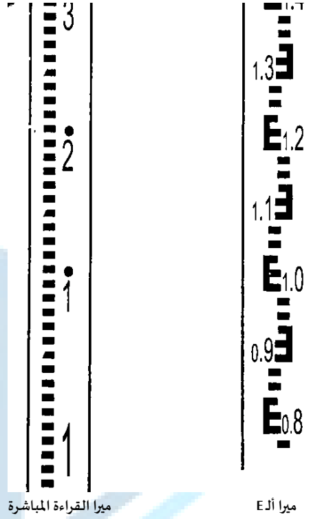
الشكل (7): ميرا التسوية.
