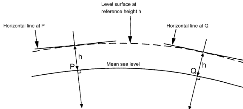
الشكل (2): تمثيل خط التسوية والخط الأفقي.
