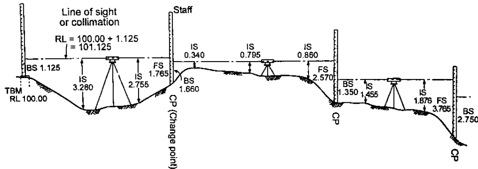
الشكل (11): التضليع الرأسي بطريقة الارتفاع عن خط الرصد.
