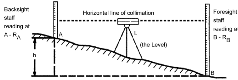
الشكل (1): الفكرة العامة للتسوية الهندسية.
