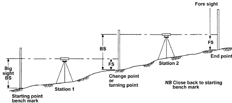
الشكل (9): تسلسل خطوات القياس ضمن المضلع الشاقولي.
