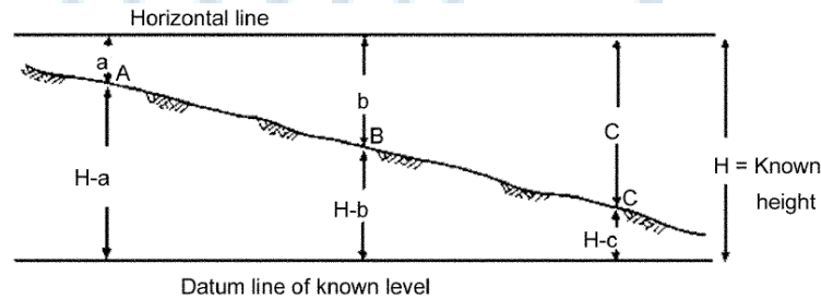
الشكل (3): الارتفاعات المختزلة للنقاط.
