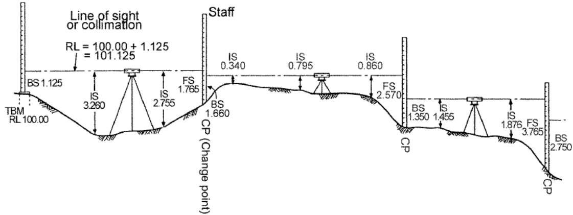
الشكل (10): كروكي المضلع الرأسى.
