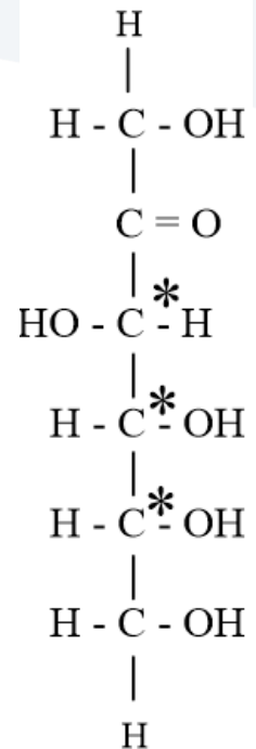
\beta -D-فركتوز
