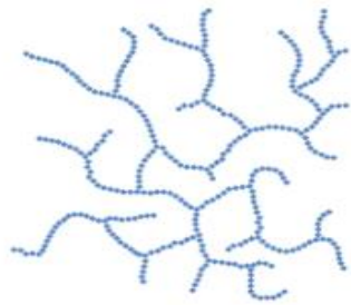
glycogen
