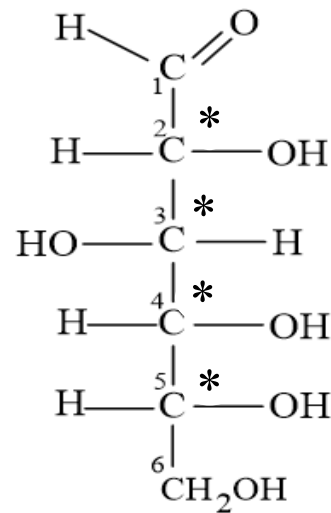
\alpha -D-غلوكوز
