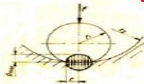
(5.2) إجهاد الهصر في كرة داخل كرة مفرغة
